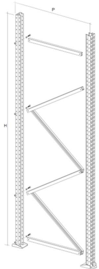
Serie L100-Z/M - spessore 20/10 Series L100-Z/M - thickness 20/10
