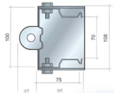
Serie L100-Z/M - spessore 20/10 Series L100-Z/M - thickness 20/10
